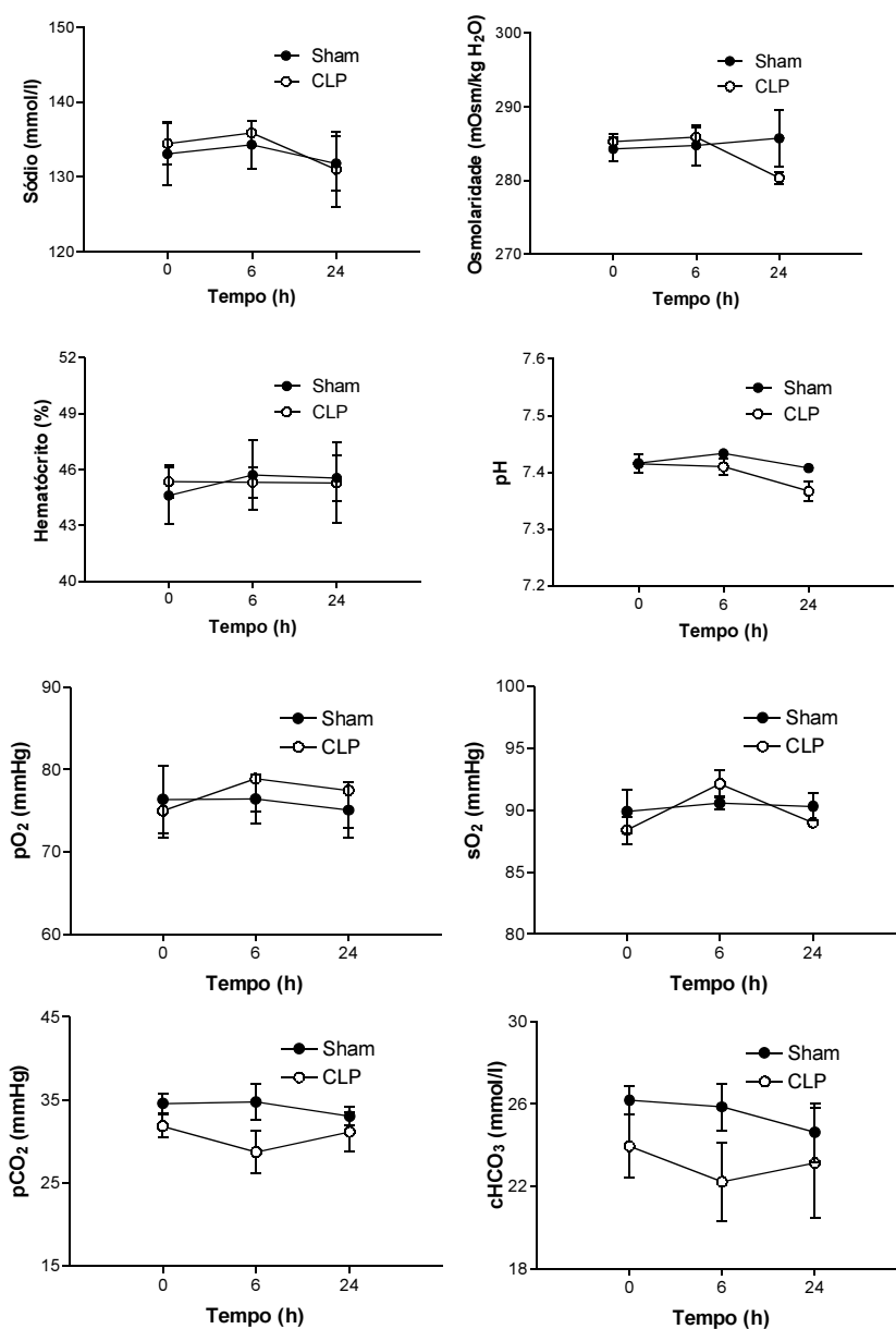
Figura 3 Concentração plasmática de Sódio, osmolaridade plasmática (mmol/l), hematócrito (%), PH, pCO 2 (mmHg), pO 2 (mmHg), sO 2 (mmHg) e cHCO 3 - (mmol/l) nos tempos 0, 6 e 24 horas após a realização da cirurgia fictícia (SHAM) ou ao CLP.
